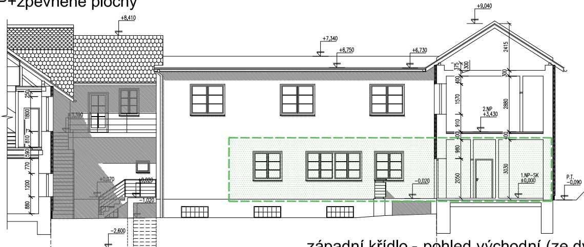
západní křídlo - pohled východní (ze dvora) s vyznačením plochy bytu, M 1:200
